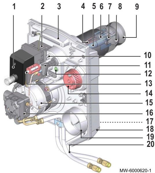
Рис.3 Основные компоненты
