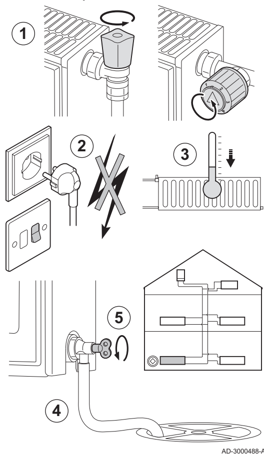
Рис.55 Слив установки
