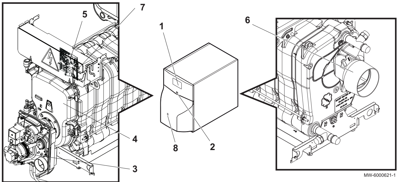
Рис.2 Основные компоненты
