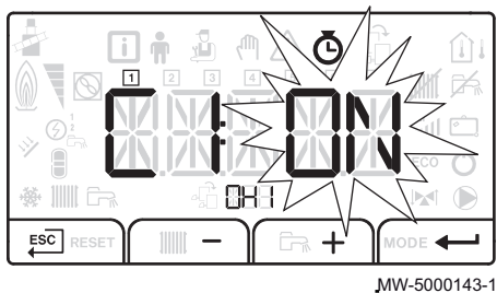
Рис.52 Выбор статуса
